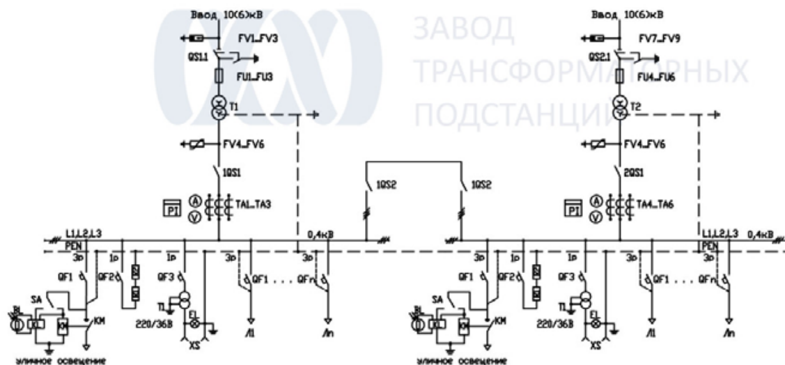
ЗКТП-ТВ(ТК) 25-400/10(6)/0,4 СХЕМА ЭЛЕКТРИЧЕСКАЯ ПРИНЦИПИАЛЬНАЯ Схема 7
