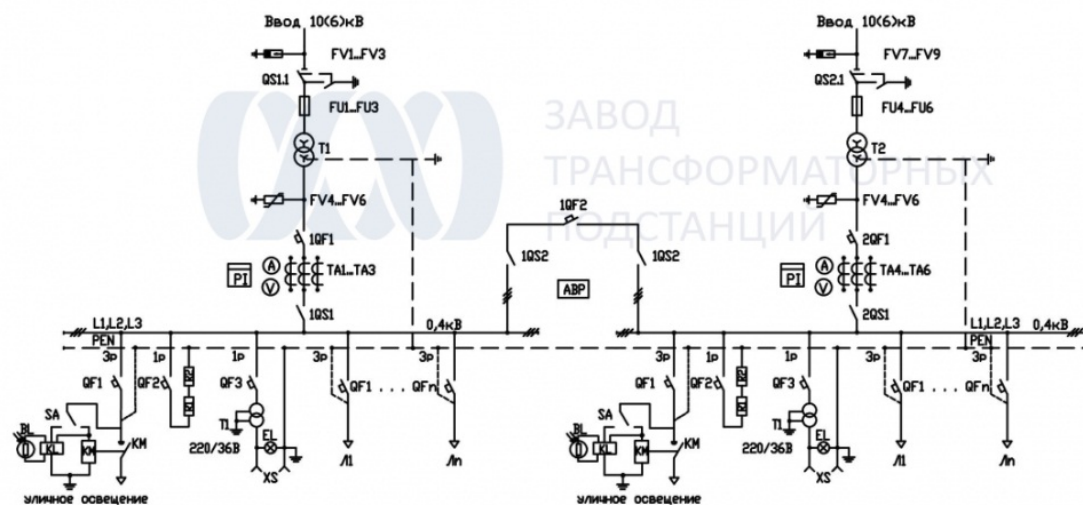
ЗКТП-ТВ(ТК) 25-400/10(6)/0,4 СХЕМА ЭЛЕКТРИЧЕСКАЯ ПРИНЦИПИАЛЬНАЯ Схема 8
