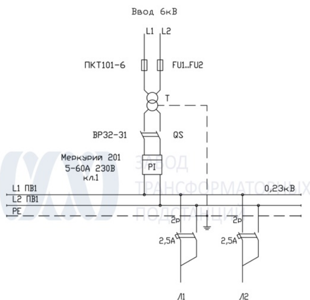
СХЕМА ЭЛЕКТРИЧЕСКАЯ ПРИНЦИПИАЛЬНАЯ Схема 5
